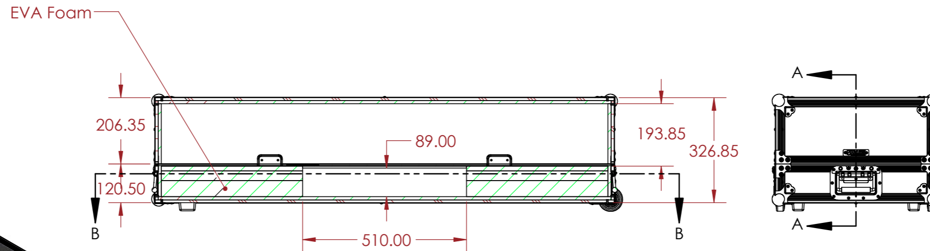
SECTION A-A
