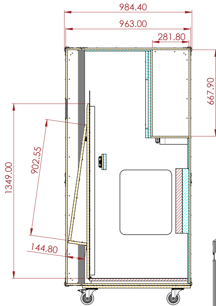
SECTION A-A SCALE 1 : 15
