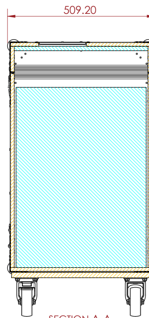
SECTION A-A SCALE 1 : 8
