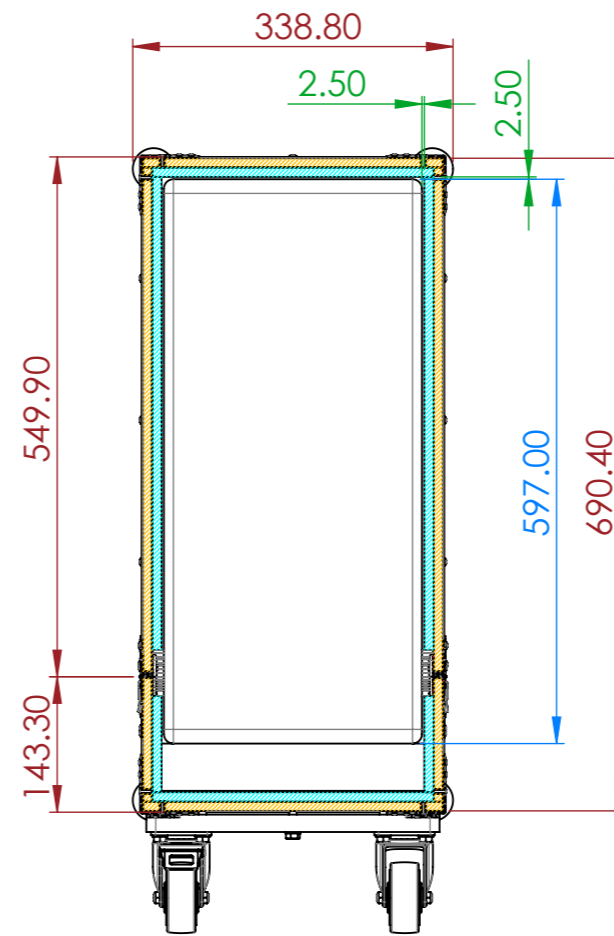
SECTION A-A
