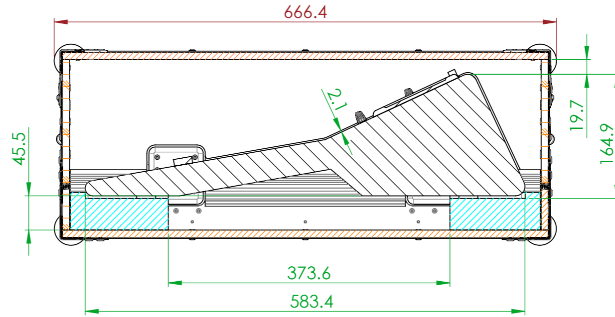
SECTION A-A
