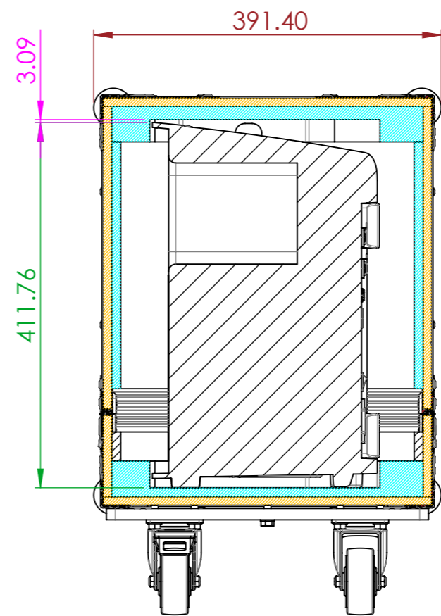
SECTION A-A SCALE 1 : 6
