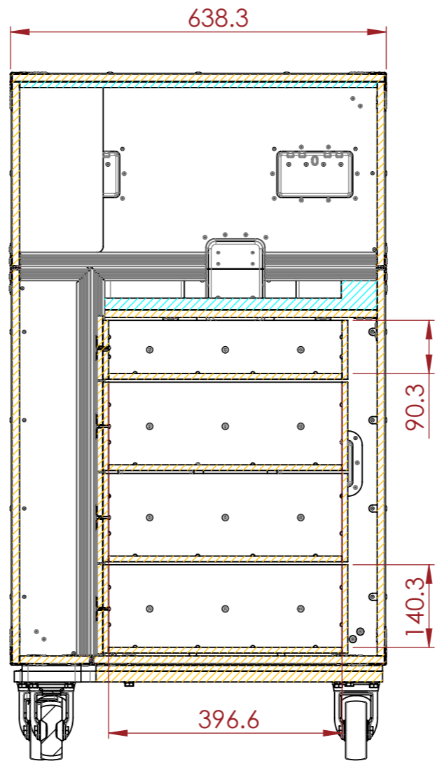
SECTION A-A
