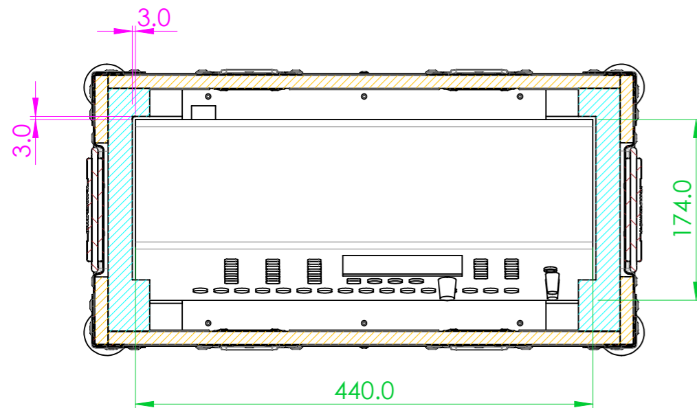
SECTION B-B SCALE 1 : 5
