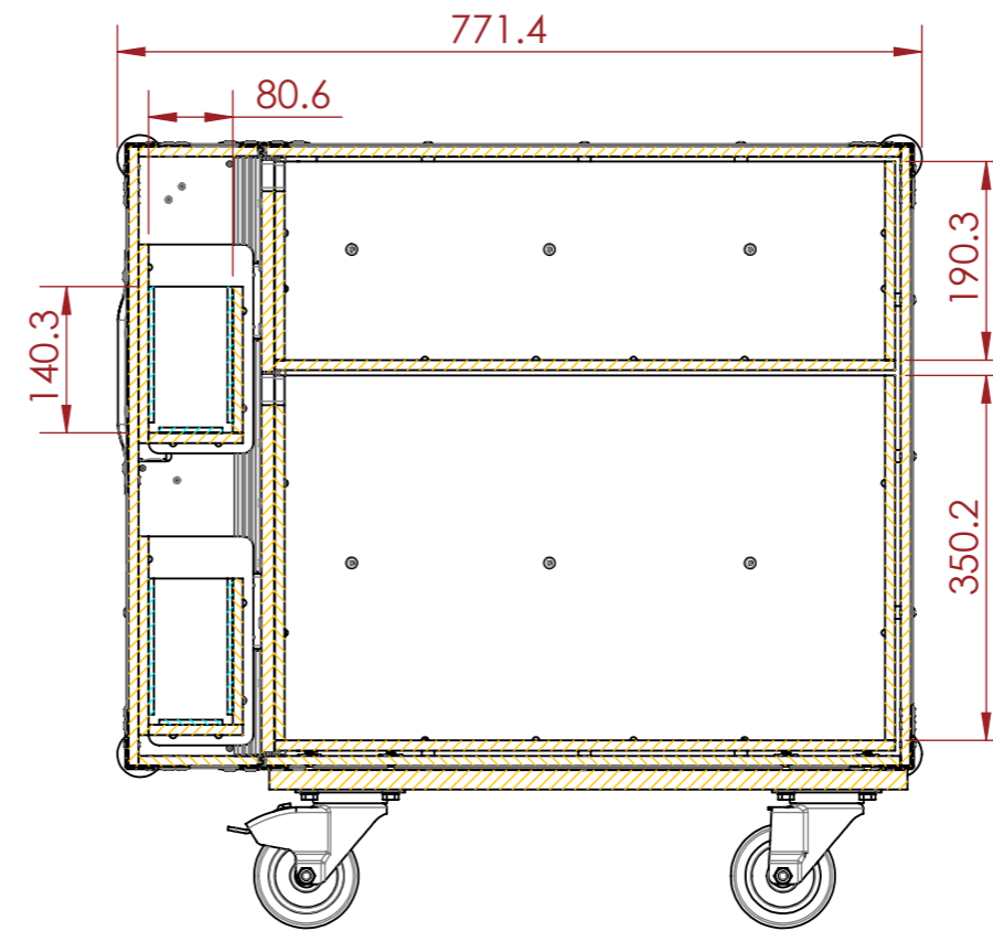
SECTION A-A SCALE 1 : 8
